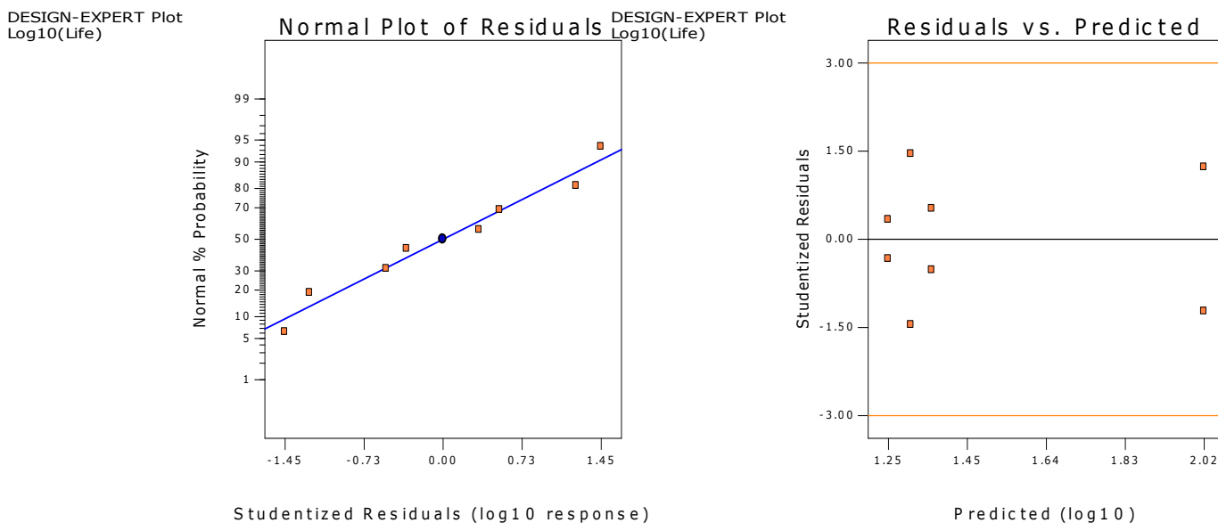
Figure 7a, b: Normal plot dei residui studentizzati e diagramma dei residui studentizzati verso i valori teorici predetti, per i dati trasformati del cuscinetto
