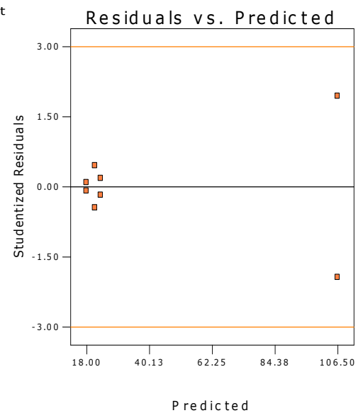
Figure 4a, b: Normal plots dei residui studentizzati e diagramma dei residui studentizzati verso i valori teorici predetti, per il caso del cuscinetto
