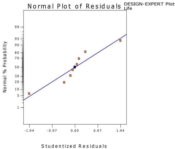
Figure 4a, b: Normal plots dei residui studentizzati e diagramma dei residui studentizzati verso i valori teorici predetti, per il caso del cuscinetto
